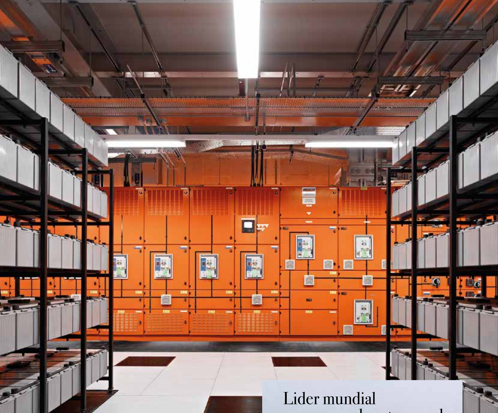
Telehouse, centro de proceso de datos (CPD). 199 unidades de ACBs TemPower2, 423 unidades de MCCBs TemBreak2.
